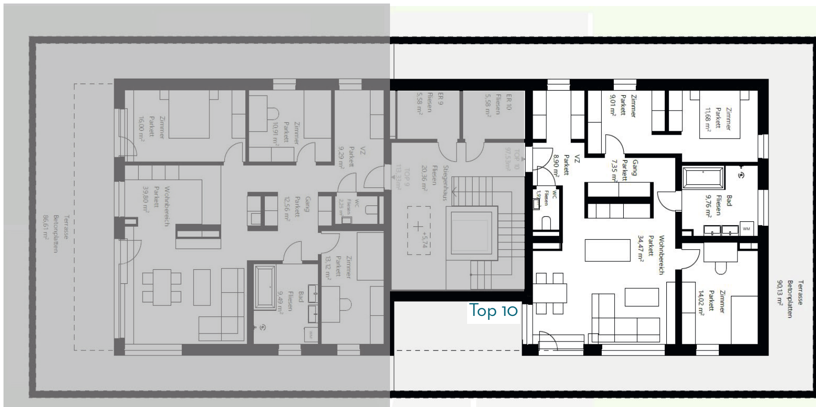
Dachgeschoss
